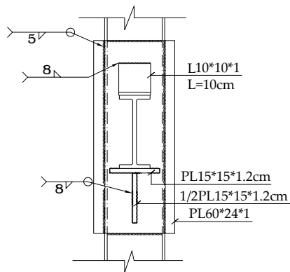
جزئیات اتصال پل به جان ستون
