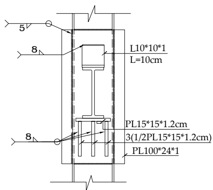
جزئیات اتصال پلهای نیروی به جان ستون
