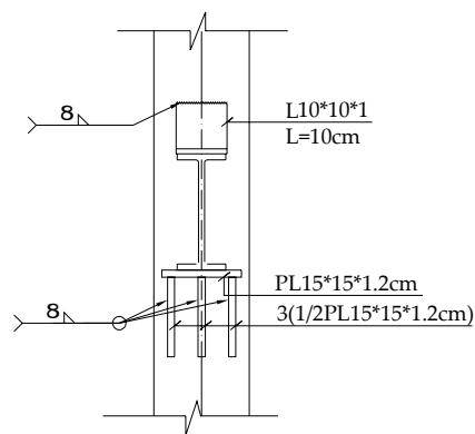
جزئیات اتصال پلهای نیروی به بال ستون
