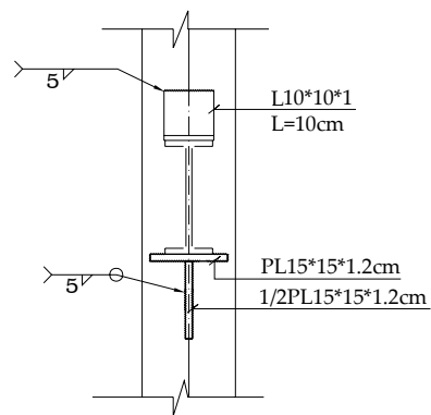
جزئیات اتصال پل به بال ستون
