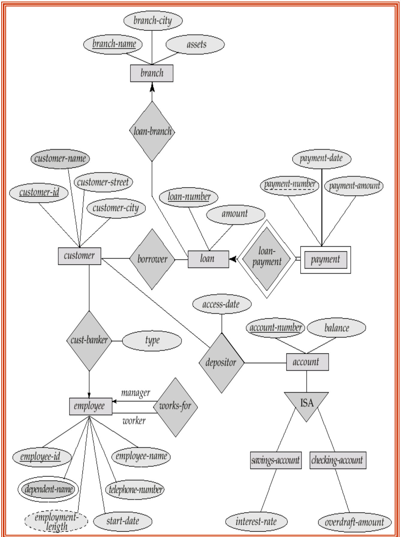
مثال : نمودار E/R یک سیستم بانکی :
