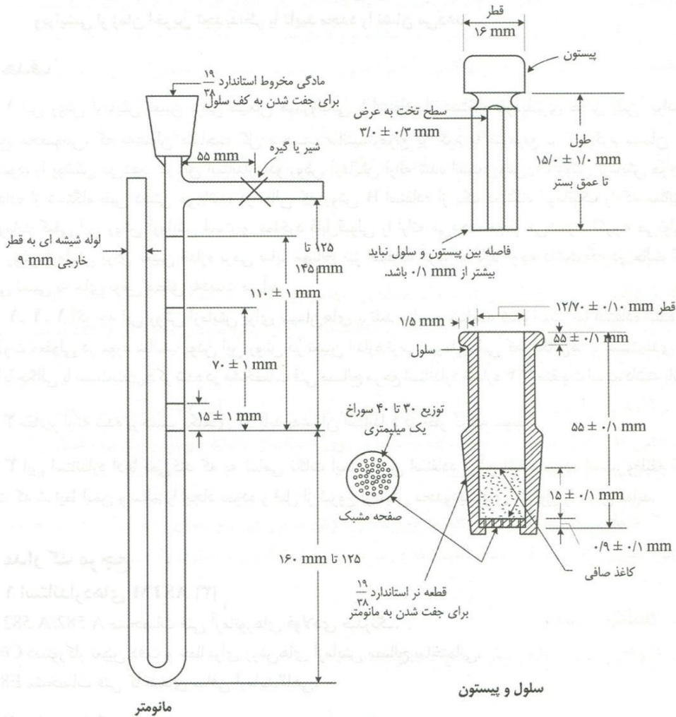
شکل ۱ دستگاه نفوذپذیری بلین.
