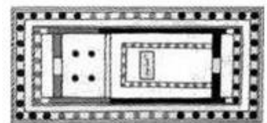
پلان معبد پارتنون
