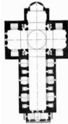
پلان کلیسای سن آندرتا
