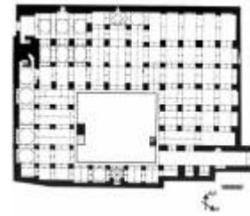
پلان مسجد جامع ناین
