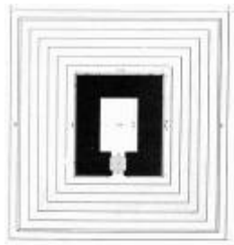
پلان آرامگاه کوروش، پاسارگاد
