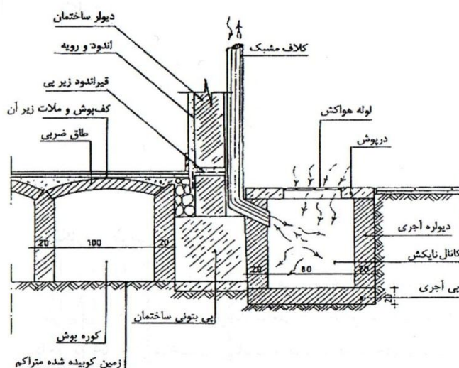
شکل ۲-۸ اجرای نایکش در اطراف خارجی ساختمان اجرای کوره
