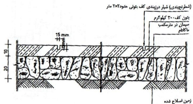
شکل ۶-۶ جزئیات کف سازی بتنی در محوطه سازی
