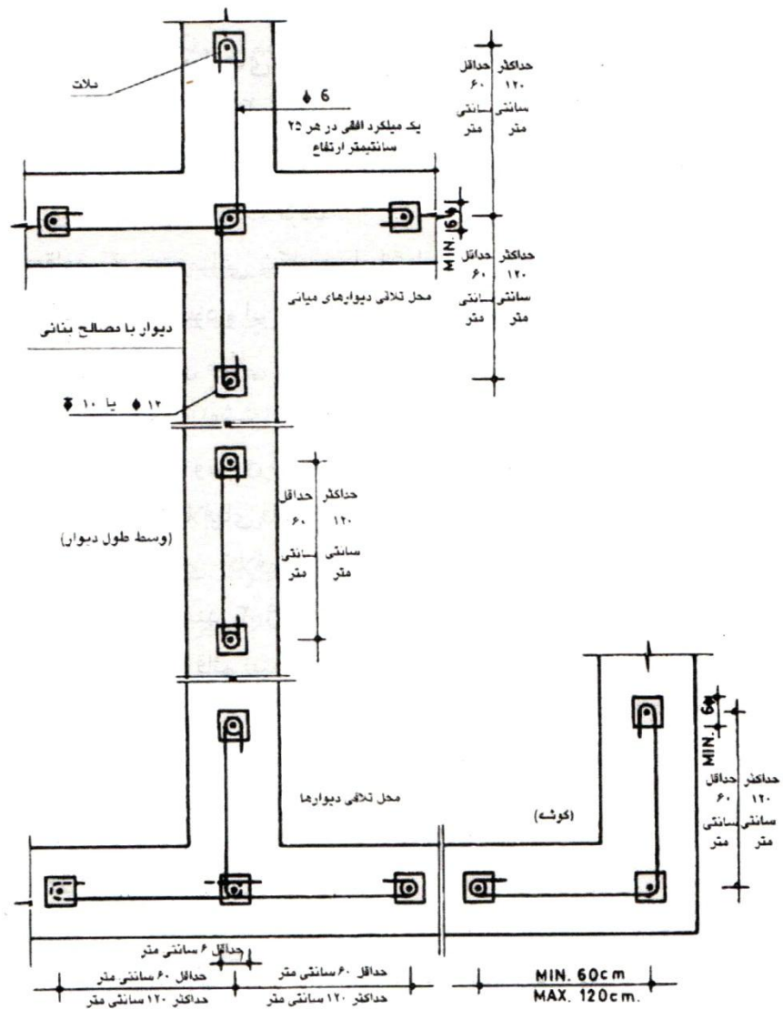
جزئیات میلگردهای قائم و افقی مهاري ديوارها
