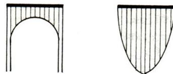
خاک چسبنده (Rigid wall) / خاک غیر چسبنده (Non-rigid wall) خطوط عمودی نشانگر شدت فشار تماس اند (Vertical lines indicate contact pressure intensity)
