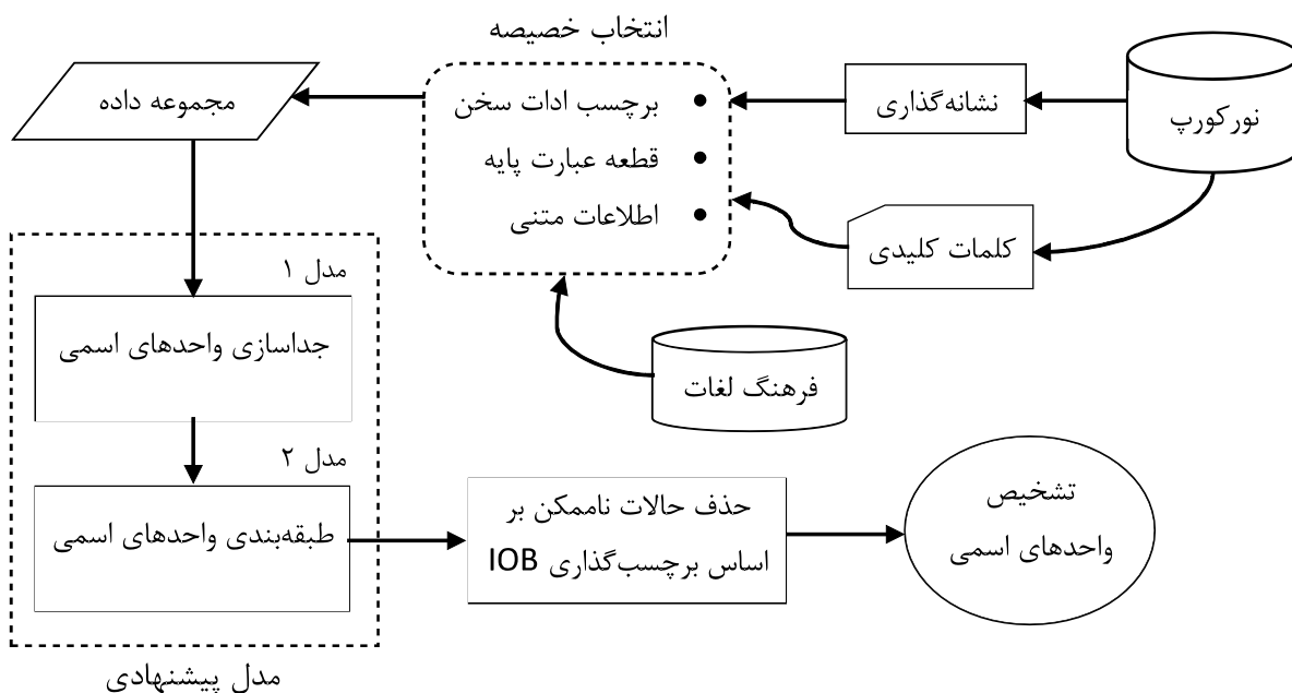
(شکل-۷): روش پیشنهادی (Figure-7): The proposal approach in detail
