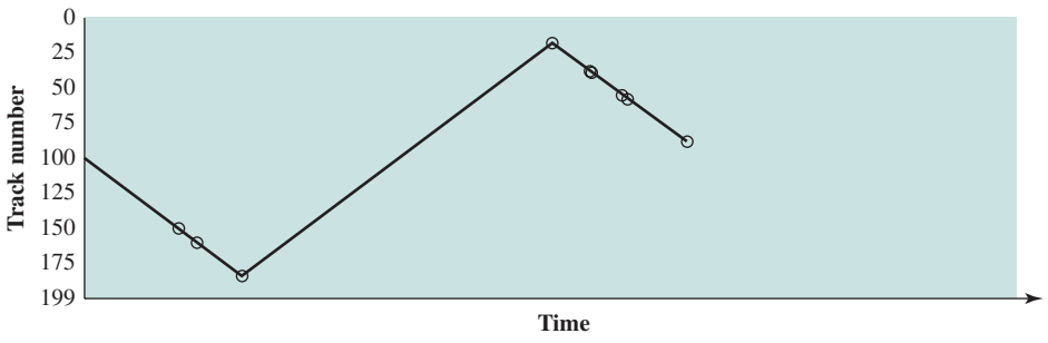
(d) C-SCAN
