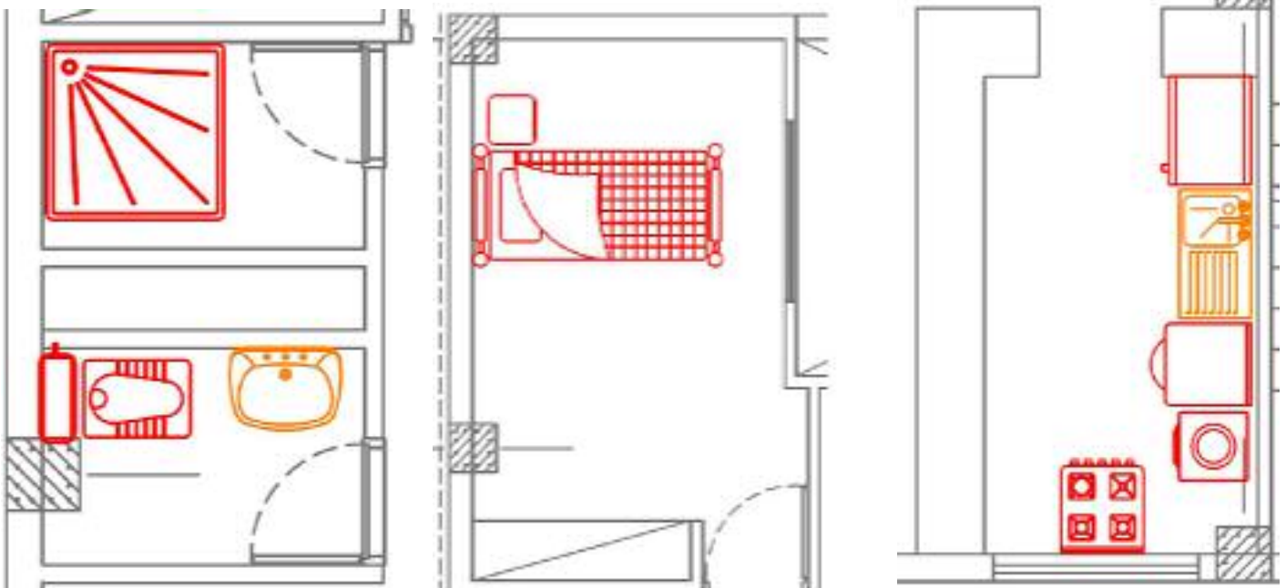
پلان حمام
