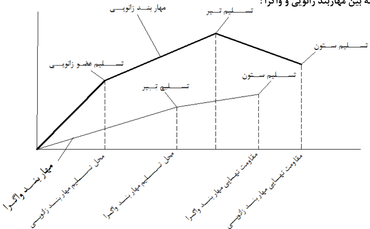
مقایسه بین مهاربند زانویی و واگرا :
