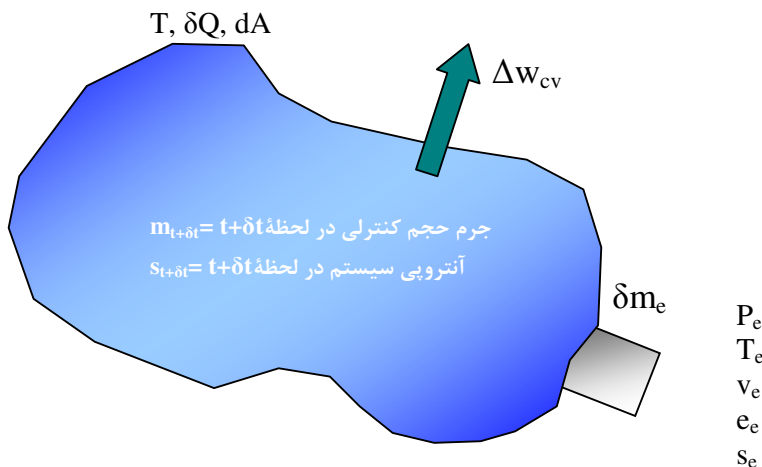
شکل ۵-۳۵. حجم کنترلی در لحظه t+δt
