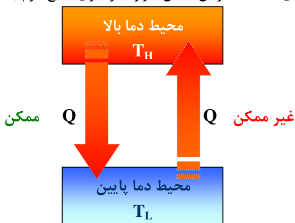
شکل ۳-۵. قانون دوم ترمودینامیک
