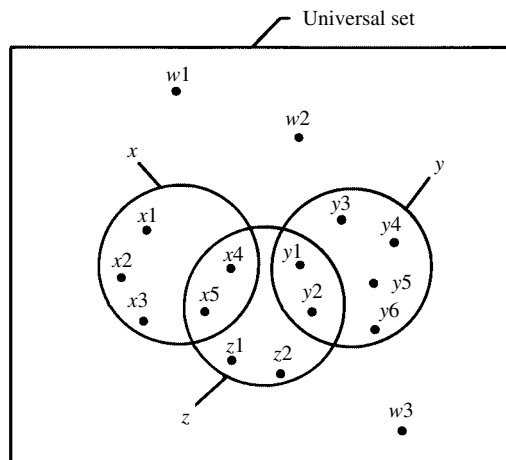
Venn diagram
