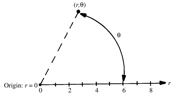
polar coordinates
