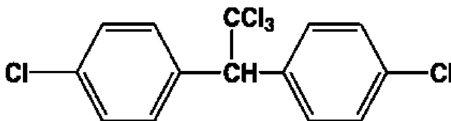
DDT
