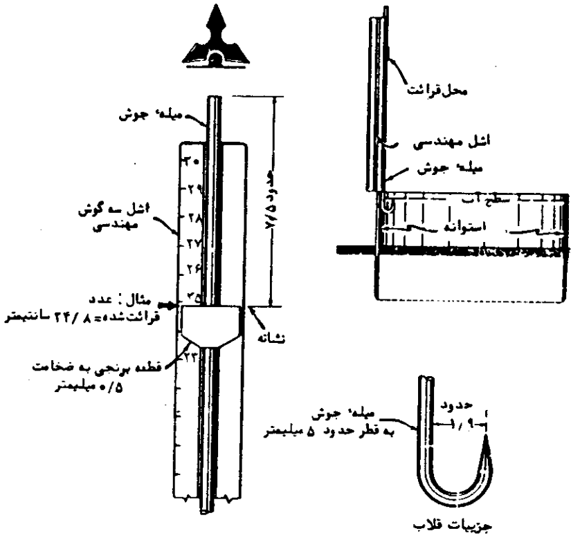
شکل ۴ - قلاب متصل به اشل مهندسی برای اندازه گیری عمق آب در استوانه
