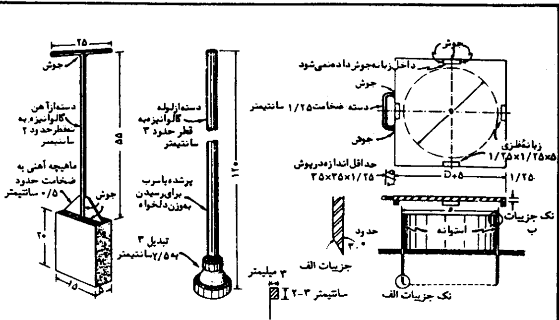
شکل ۲ - استوانه فلزی و درپوش جزئیات ب شکل ۳ - دو نوع چکش جزئیات الف
