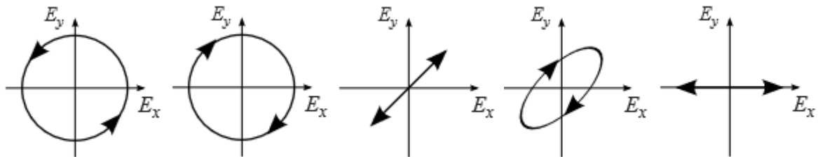
شکل ۶-۲ انواع پلاریزاسیون‌های خطی، دایروی و بیضوی [10]
