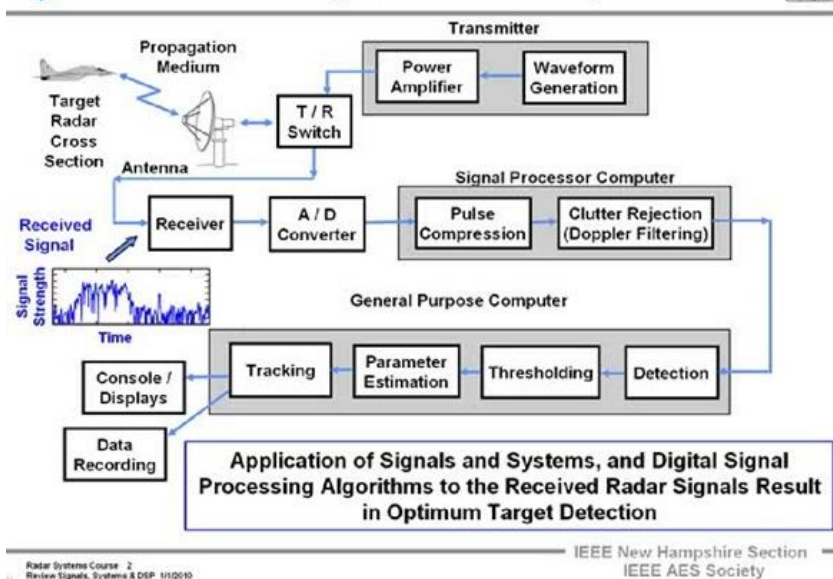
شکل ۳-۱ - شما کلی از سیستم رادار پالسی [2]
