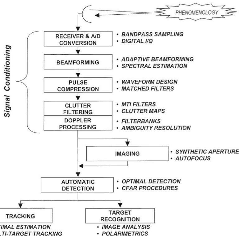
شکل ۲-۱ کلیت پردازش سیگنال در رادار [1]
