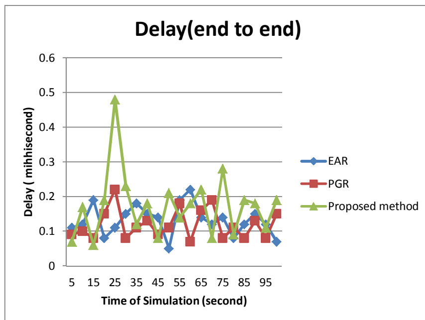
نمودار ۴-۵ تاخیر انتها به انتها به انتهای شبکه
