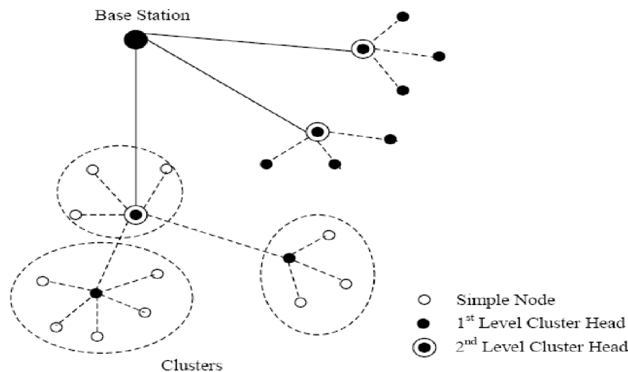
شکل ۲-۱۰ پروتکل TEEN [۵]
