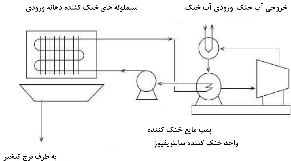
شکل ۲ - شماتیک یک سیستم خنک کننده هوای دهانه ورودی توربین
