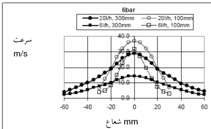
شکل ۱۱: مقایسه بین مقادیر سرعت و توزیع سرعت بر حسب شعاع افشانک برای افشانک های شماره ۲۱ و
