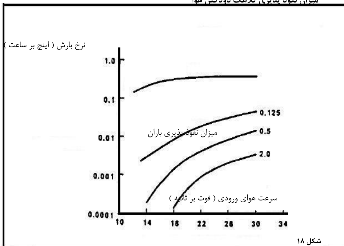
میزان نفوذ پذیری کلاهک دودکش هوا
