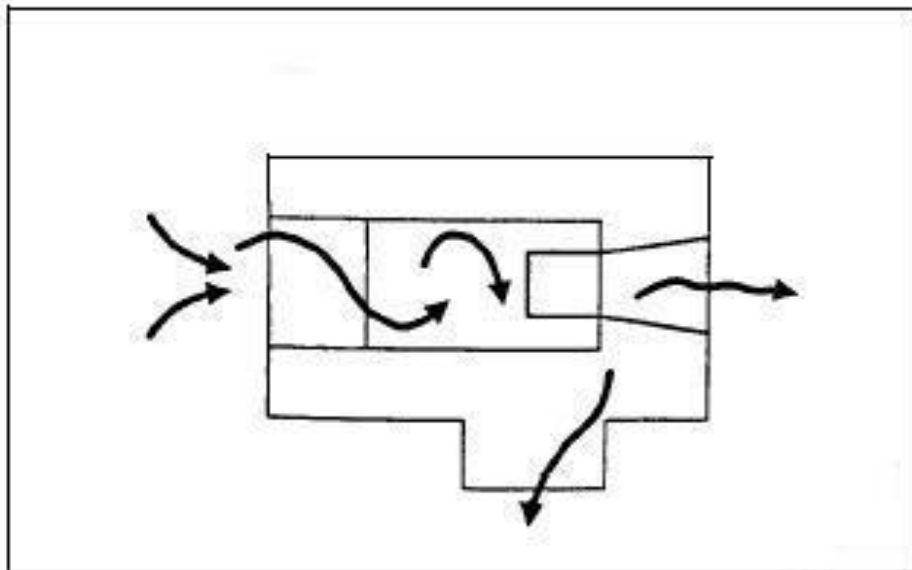
فیلتر اینرسی(ساکن)از نوع فرفرهای (چرخشی)
