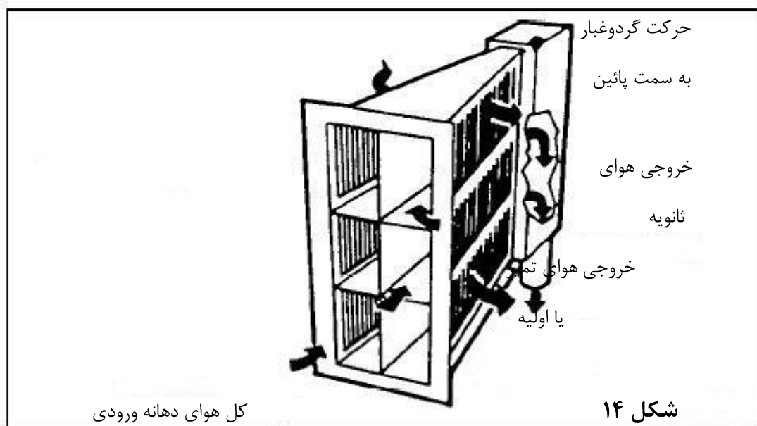
فیلتر اینرسی (ساکن) از نوع پره ای
