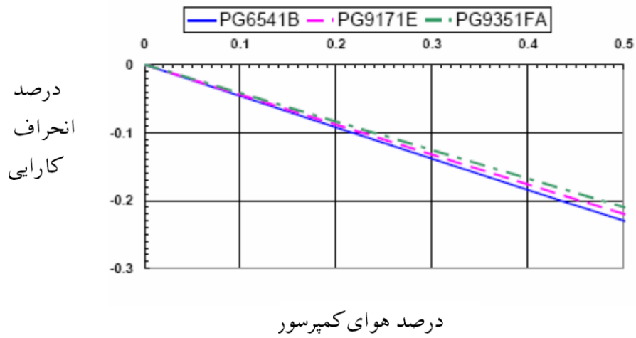
شکل ۱۶: چگونگی تاثیر هوا در کاهش کارایی توربین گازی
