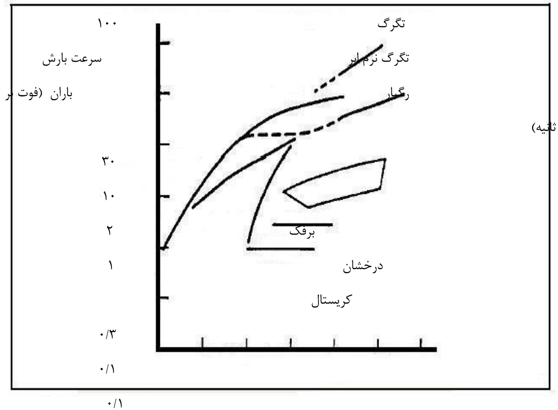
سرعت نهایی بارش با شکل‌های مختلف
