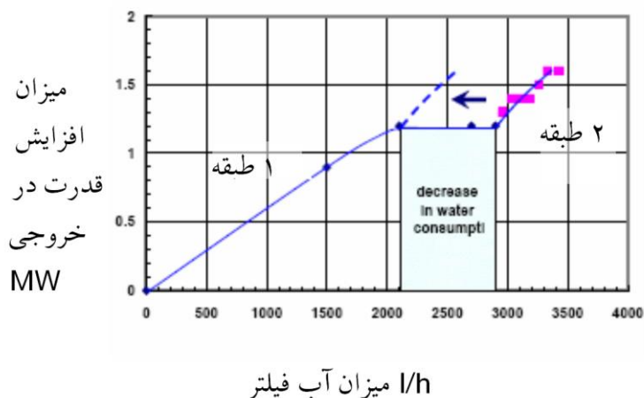
شکل ۲۲: کارایی سیستم افزایش دهنده برق دو طبقه
