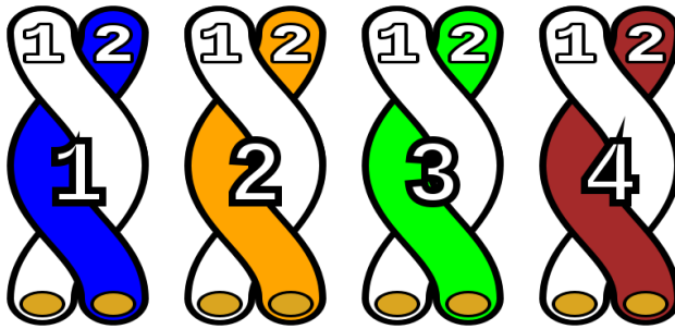
شکل ۳-۷: ساختار سیم کشی زوج بهم تابیده
