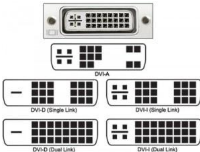
شکل ۲-۳۱: انواع درگاه های DVI
