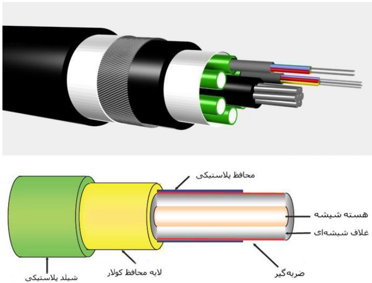
شکل ۳-۵: نمایی از فیبرنوری و ساختار آن
